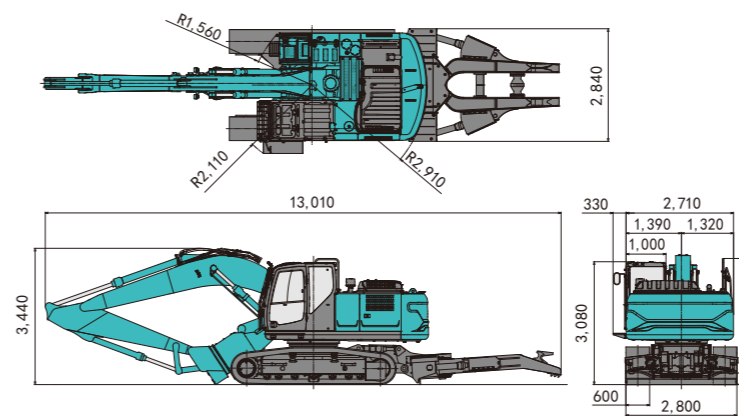
SK210D多功能解体机
