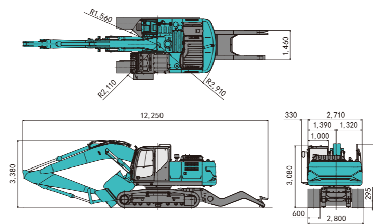
SK210D多功能解体机
